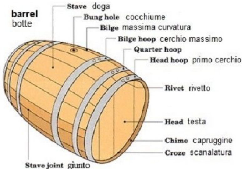
Botte in legno e sue parti (fonte http://macosa.dima.unige.it/diz/b4/botte.htm )
