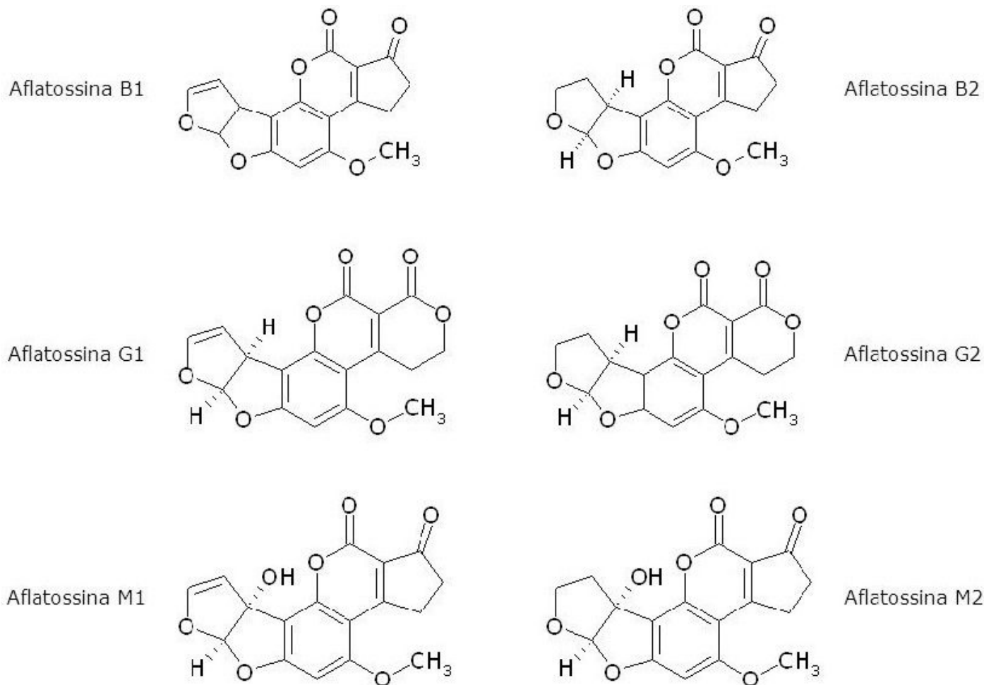
Famiglia delle Aflatossine (struttura chimica).
